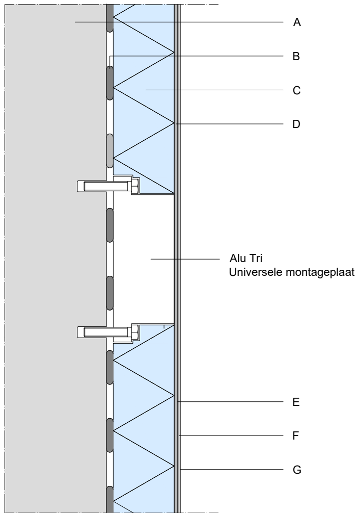
Principedetail: Doorsnede aansluiting Alu Tri montageblok
