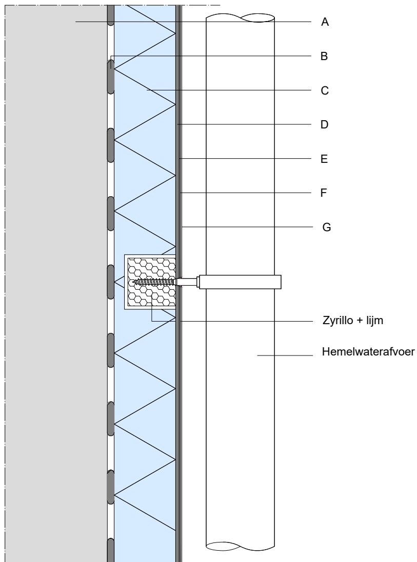
Principedetail: Doorsnede hemelwaterafvoeren met Zyrillo
